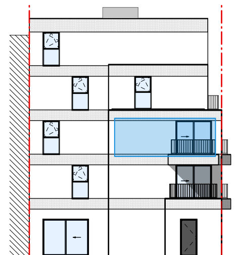
LINKER ZIJGEVEL
